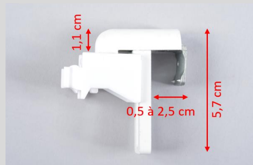
Détail et dimensions du support
