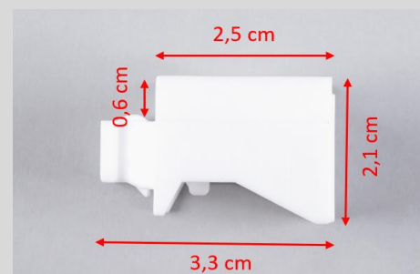
Détail et dimensions du support
