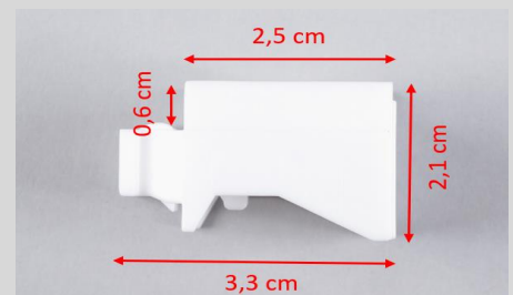
Détail et dimensions du support
